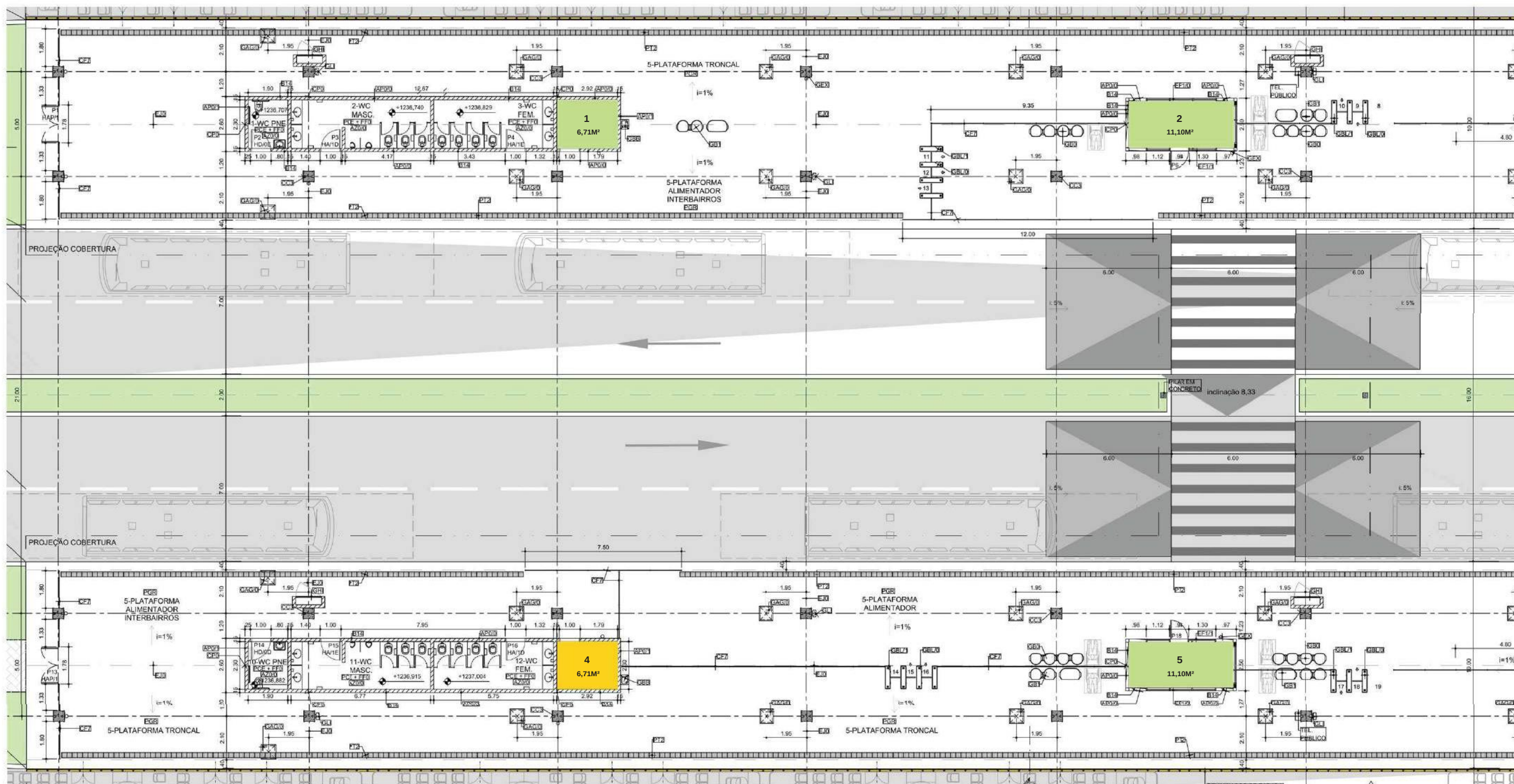
TERMINAL BRT SUL SANTA MARIA - PLANTA 1
