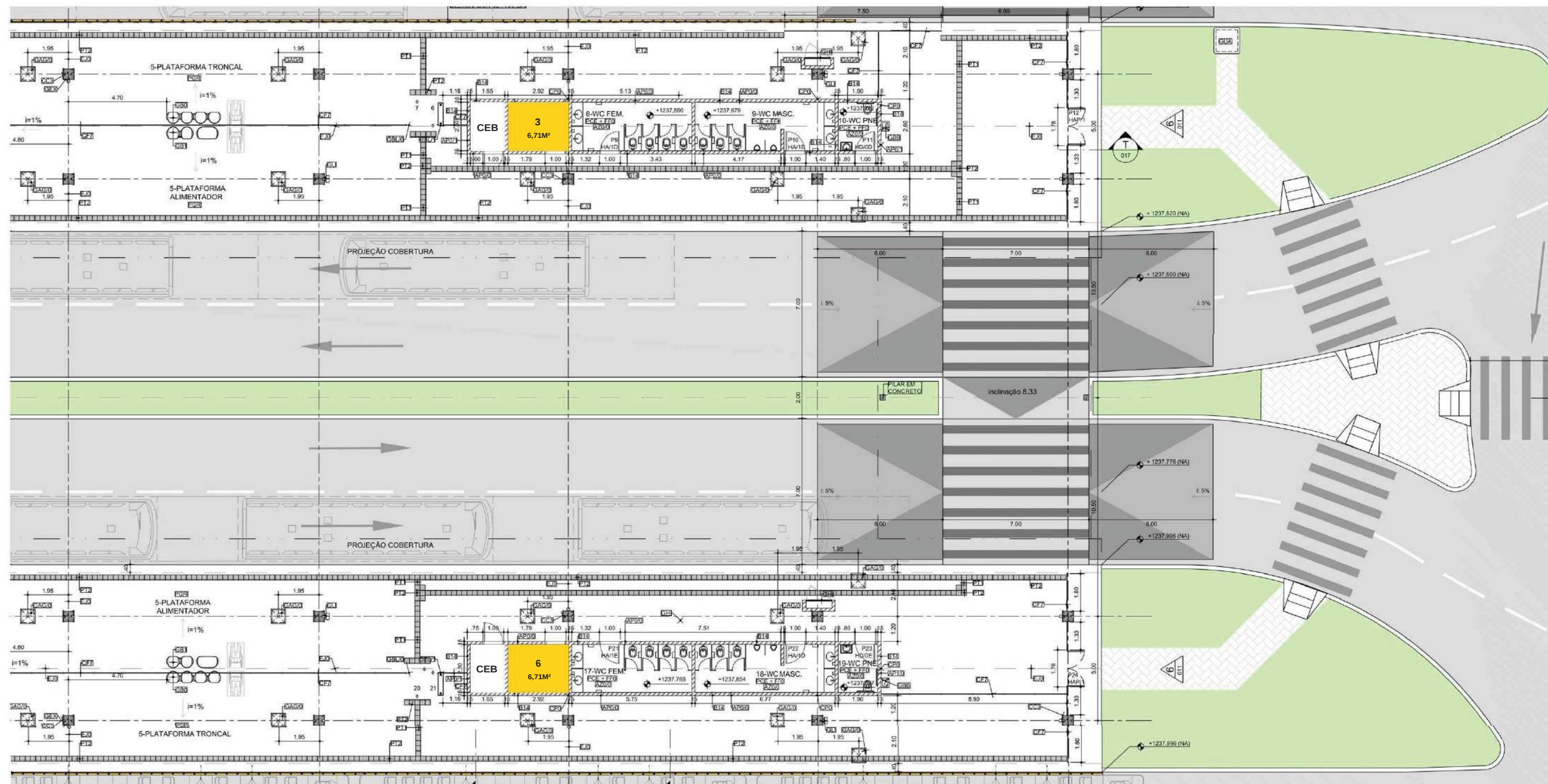
TERMINAL BRT SUL SANTA MARIA - PLANTA 2
