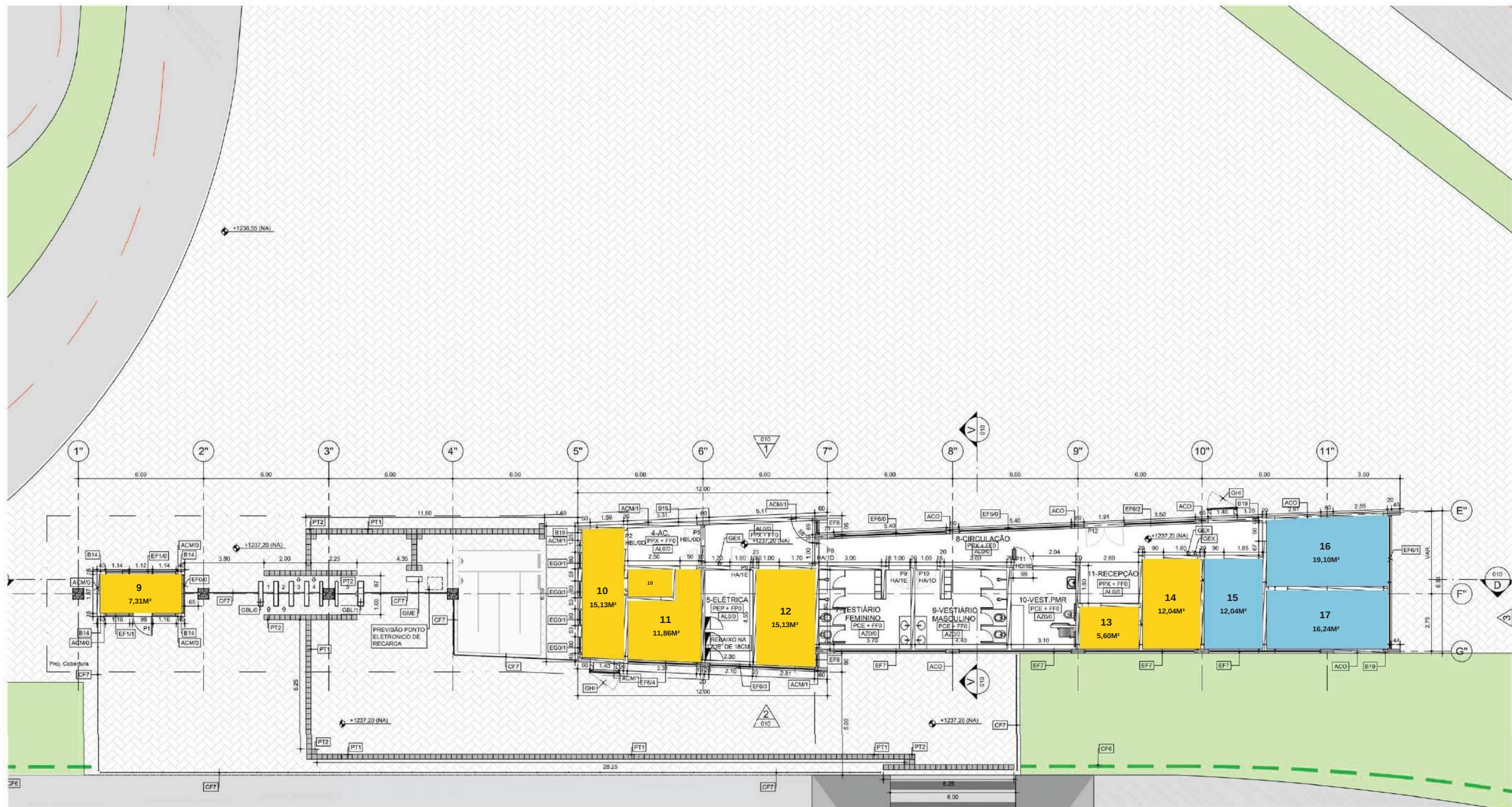
TERMINAL BRT SUL SANTA MARIA - PLANTA 4
