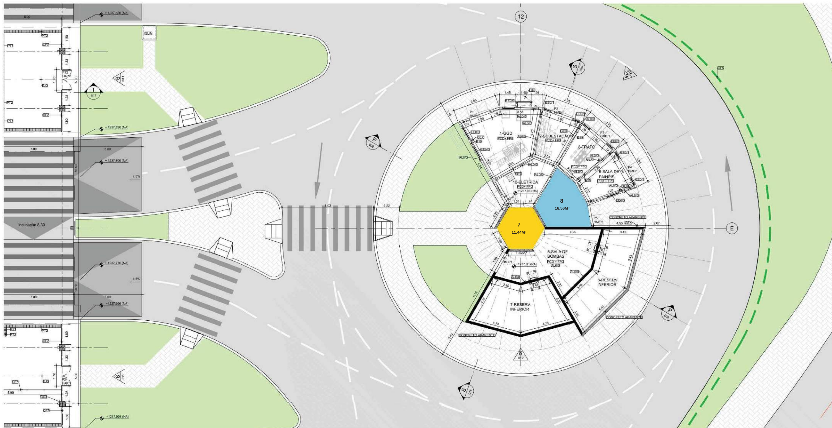
TERMINAL BRT SUL SANTA MARIA - PLANTA 3
